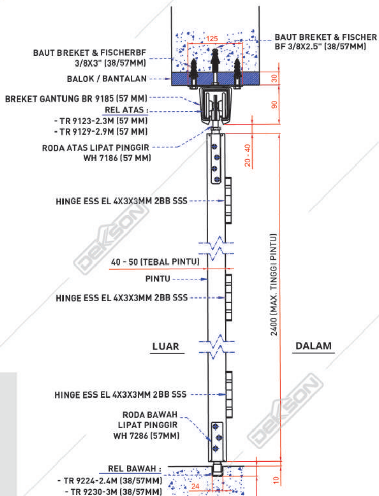
Gambar Potongan
