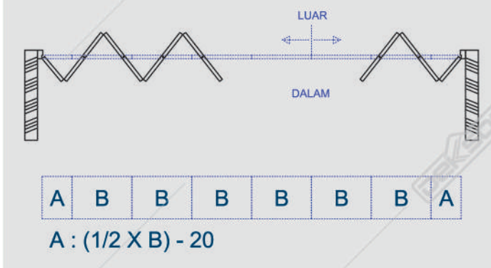
Gambar Tampak Atas
