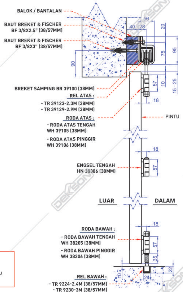
Gambar Potongan
