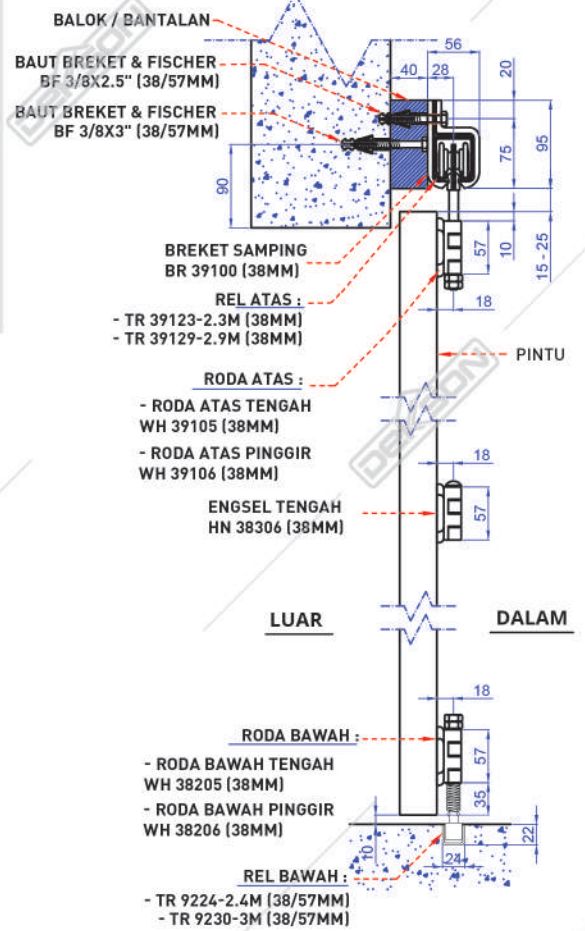
Gambar Potongan
