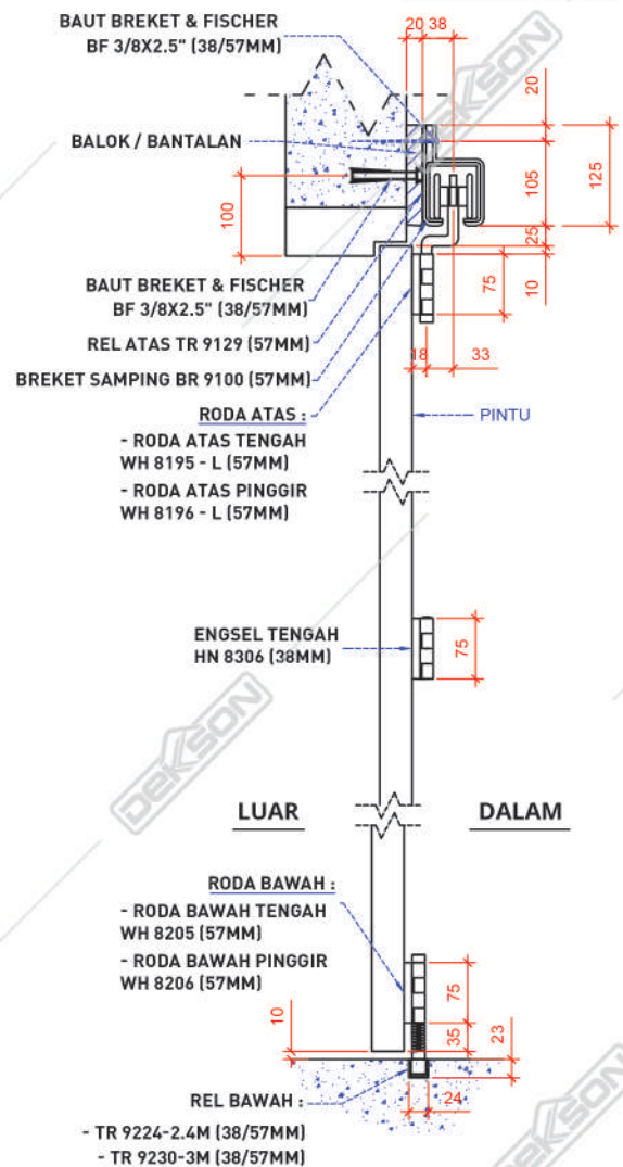
Gambar Potongan
