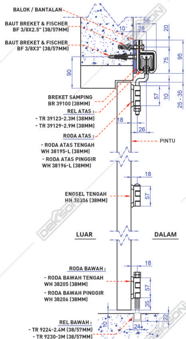
Gambar Potongan
