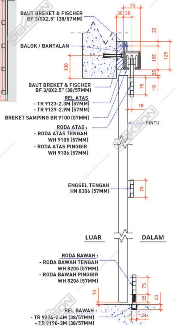
Gambar Potongan
