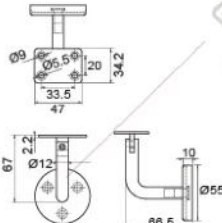
SCH 0312 RW STRAIGHT SSS Available: SCH 0312 RW OVAL SSS
