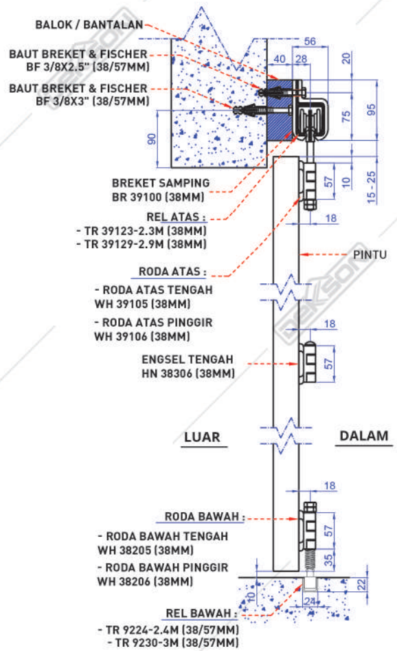
Gambar Potongan
