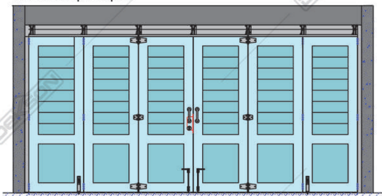
Gambar Tampak Depan
