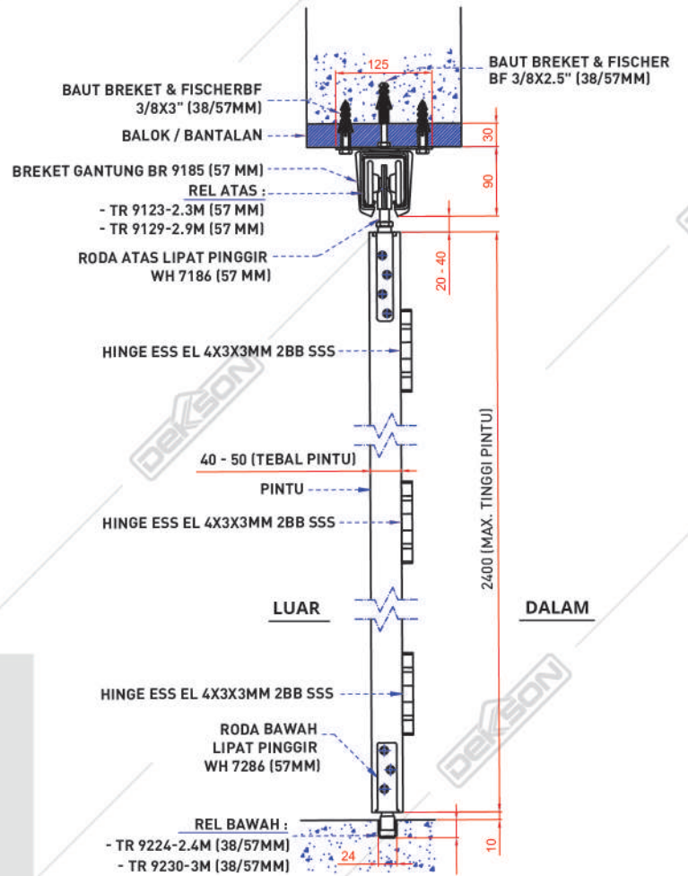
Gambar Potongan
