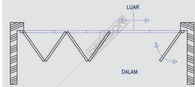
Gambar Tampak Atas
