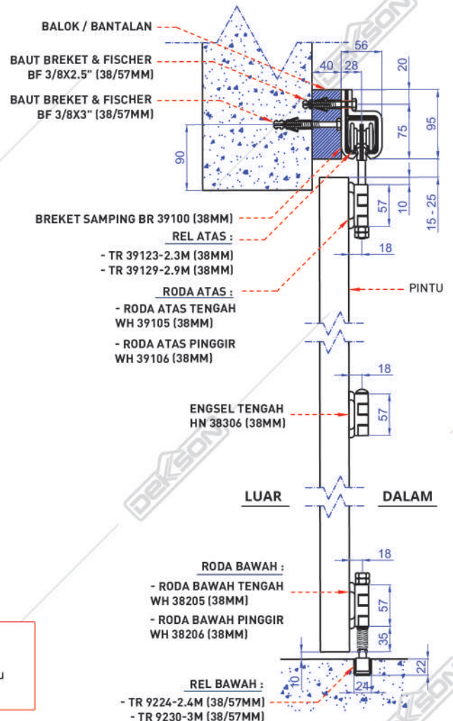
Gambar Potongan
