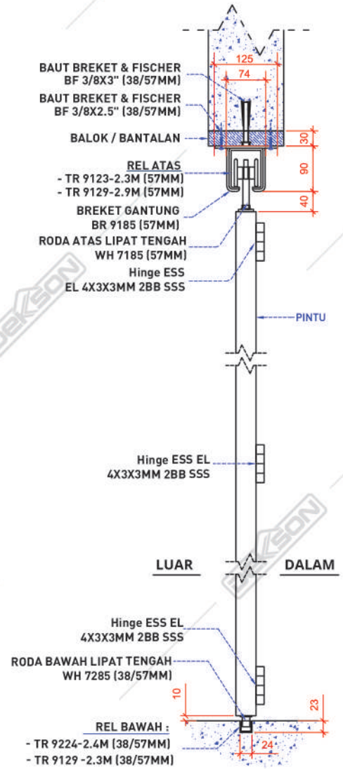
Gambar Potongan
