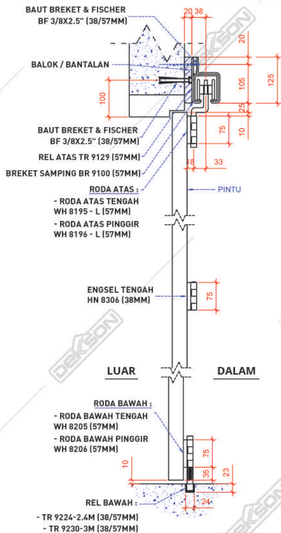
Gambar Potongan
