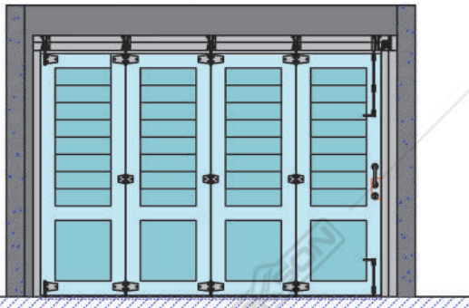
Gambar Tampak Depan
