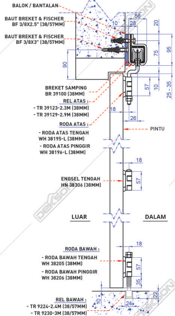
Gambar Potongan
