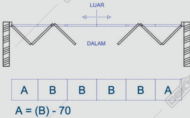
Gambar Tampak Atas
