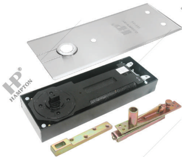
FH 84 SSS Max Capacity : 80 kg Max Door Width : 900 mm
