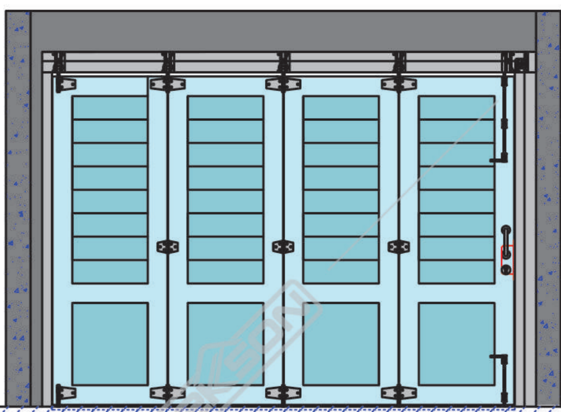
Gambar Tampak Depan
