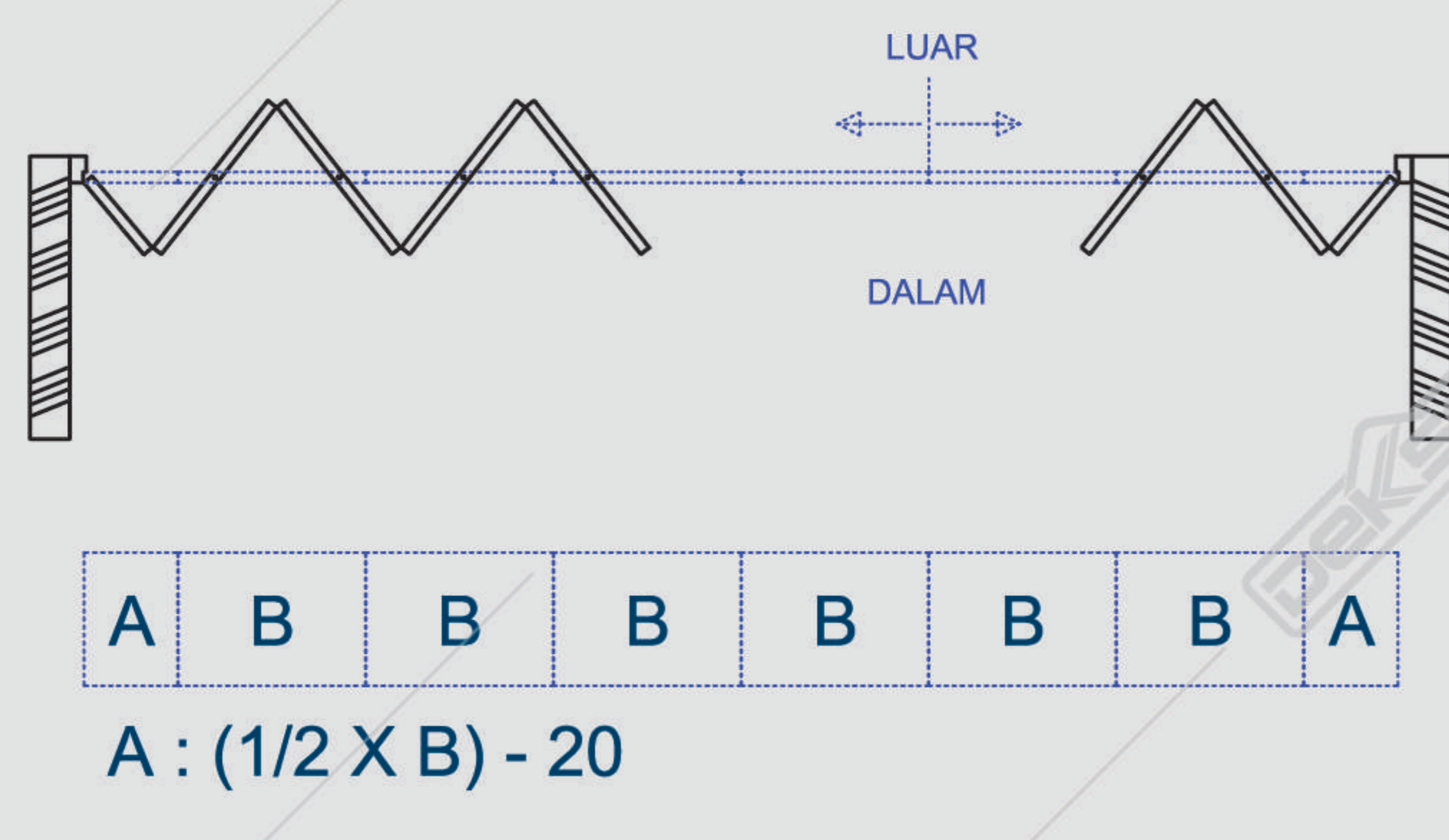
Gambar Tampak Atas
