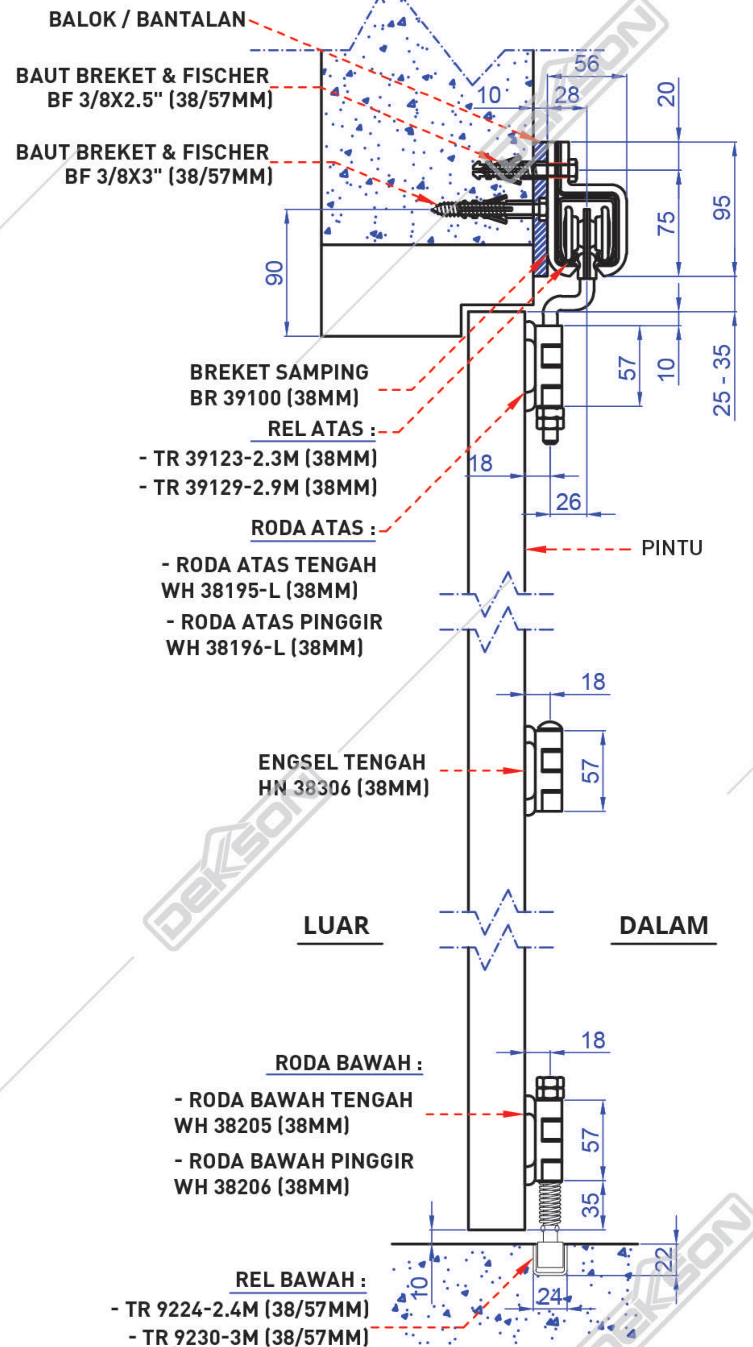
Gambar Potongan
