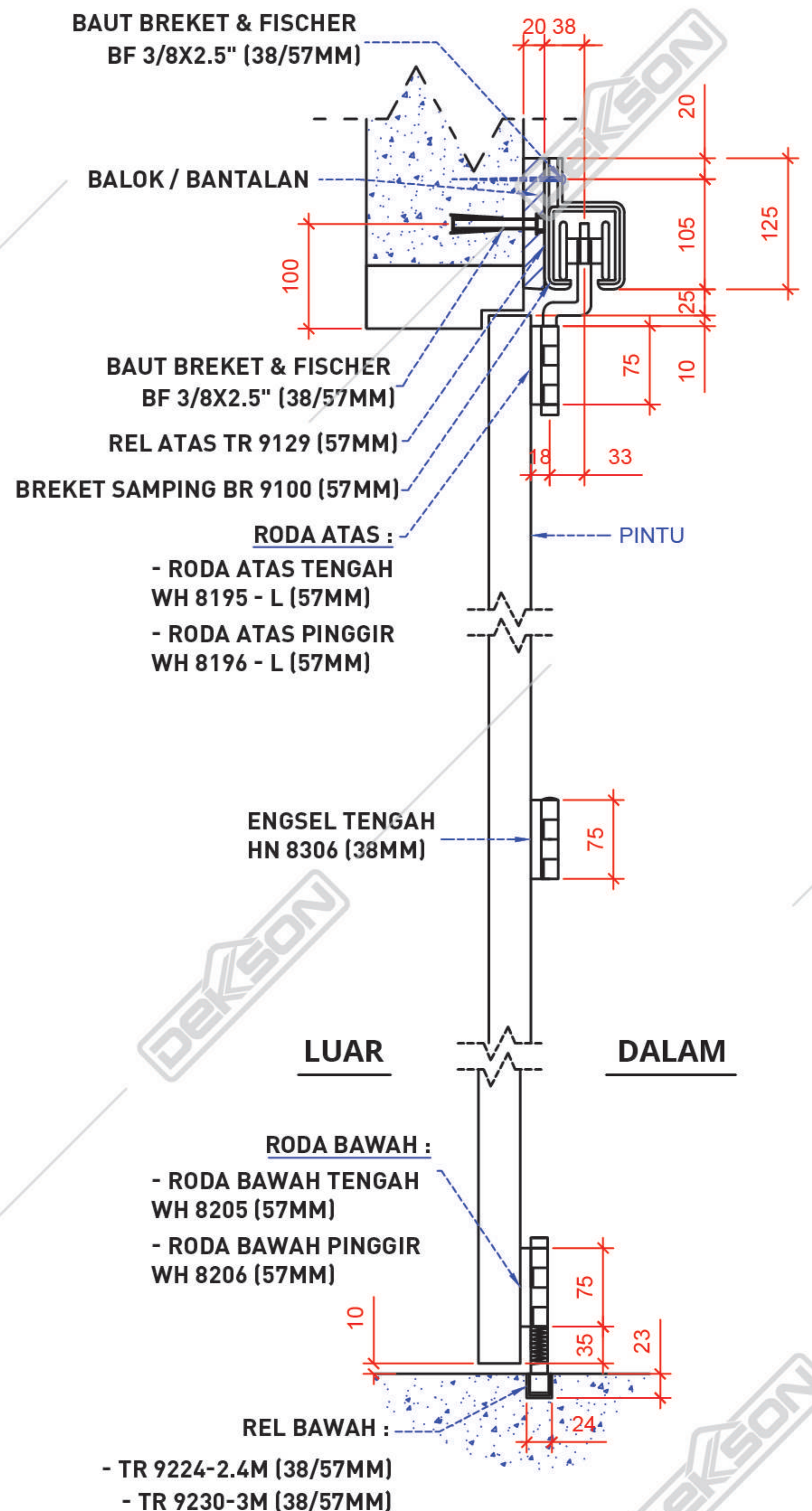
Gambar Potongan
