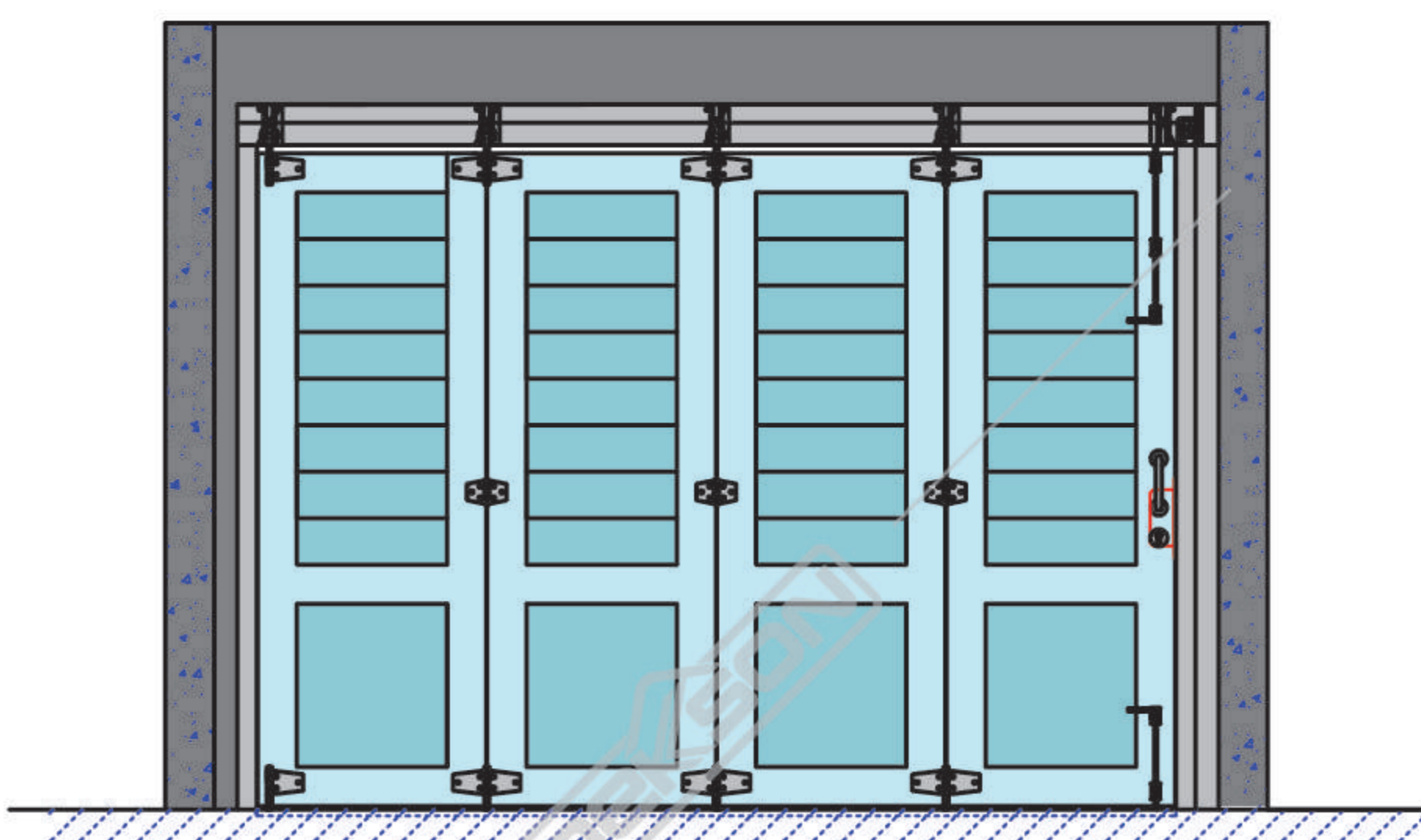
Gambar Tampak Depan
