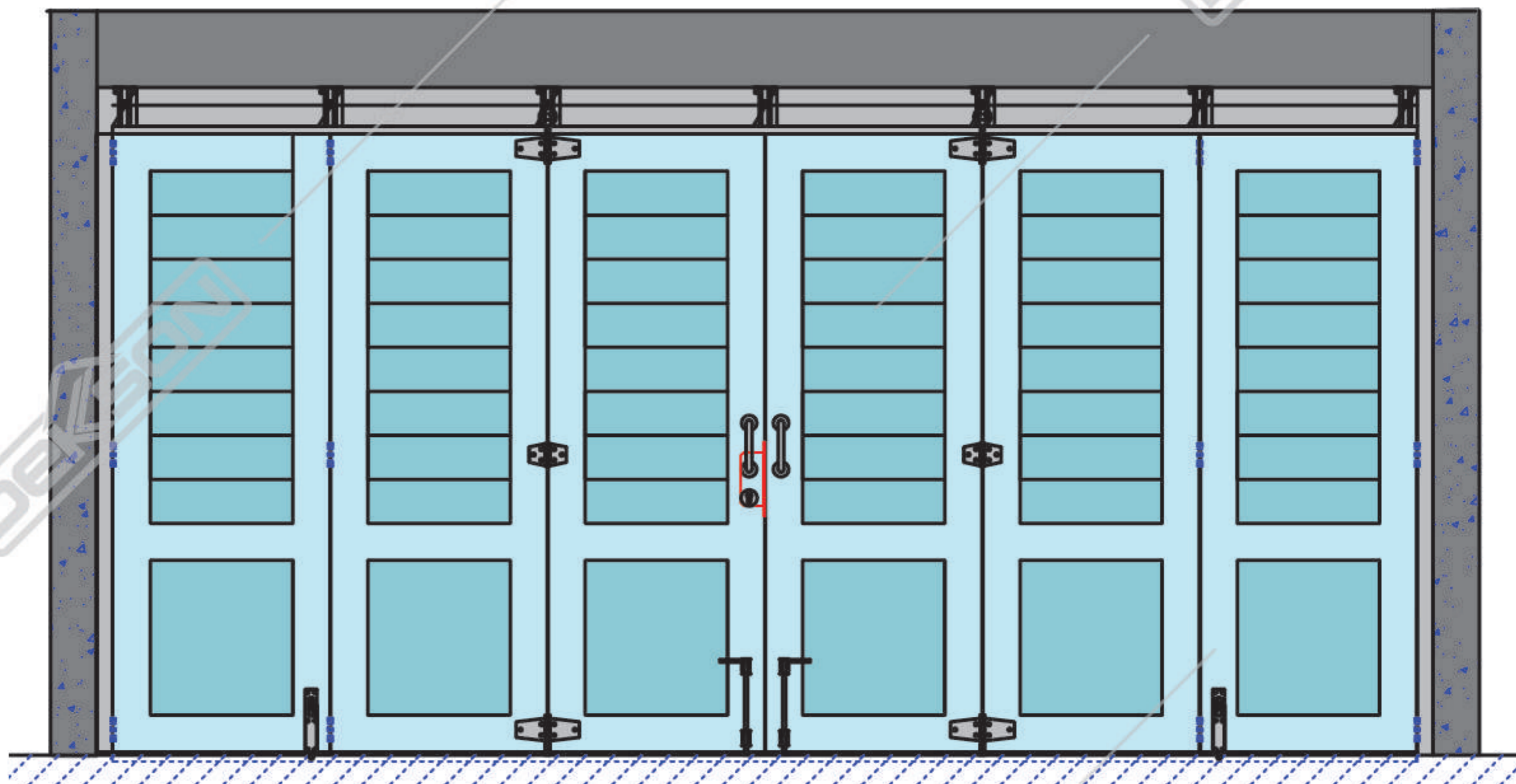
Gambar Tampak Depan
