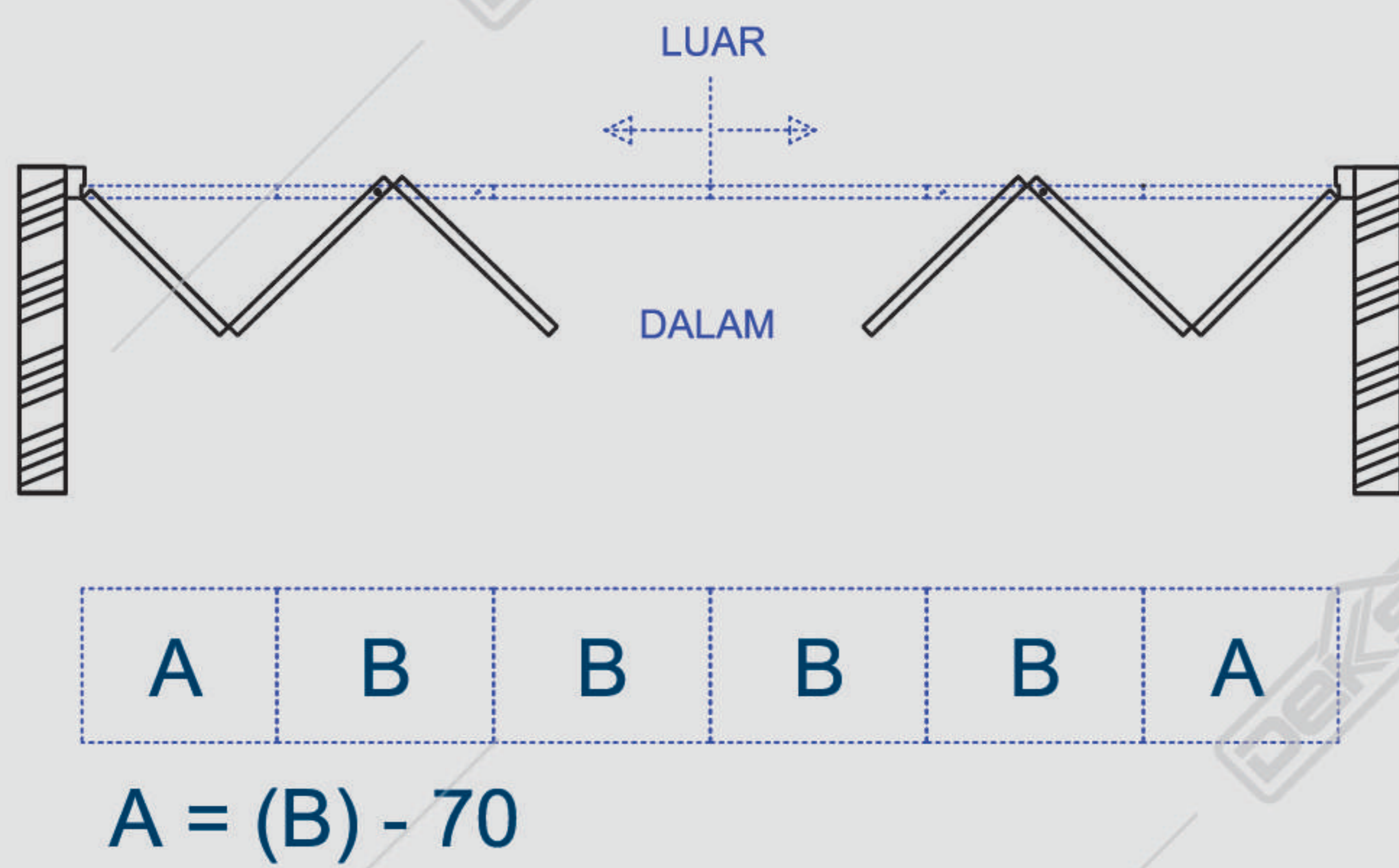
Gambar Tampak Atas
