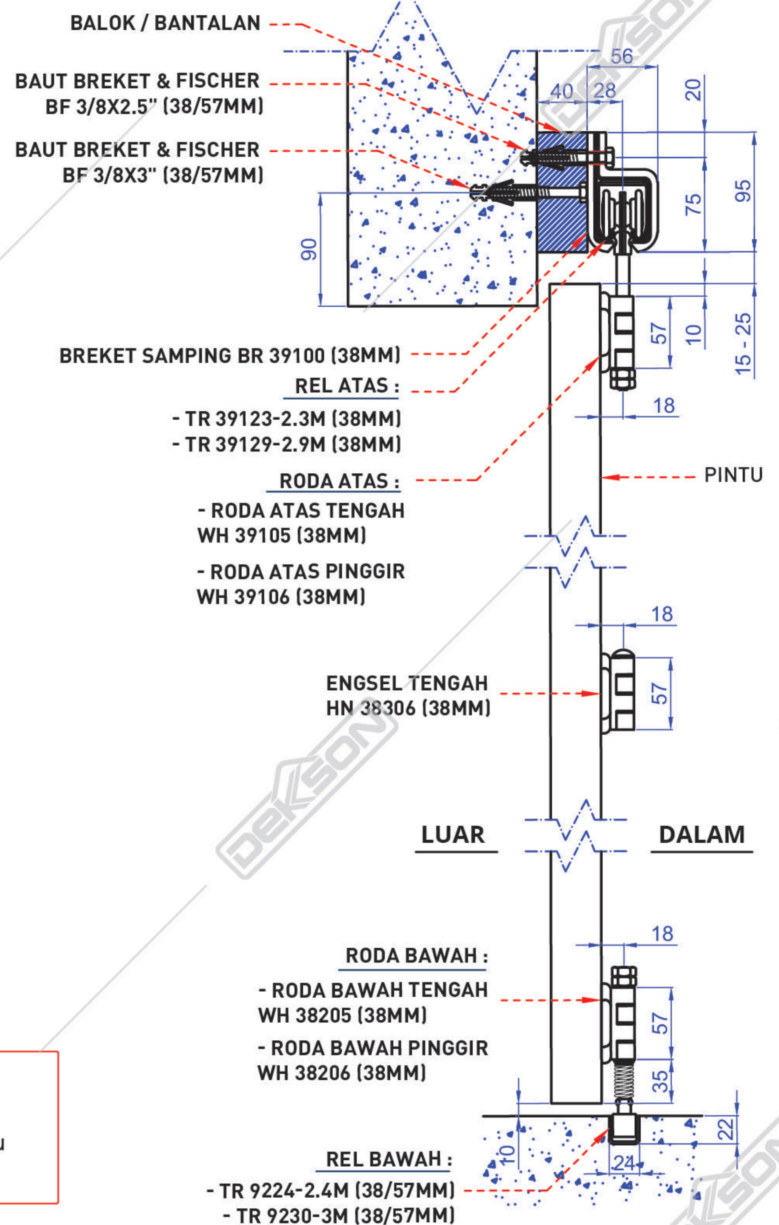
Gambar Potongan
