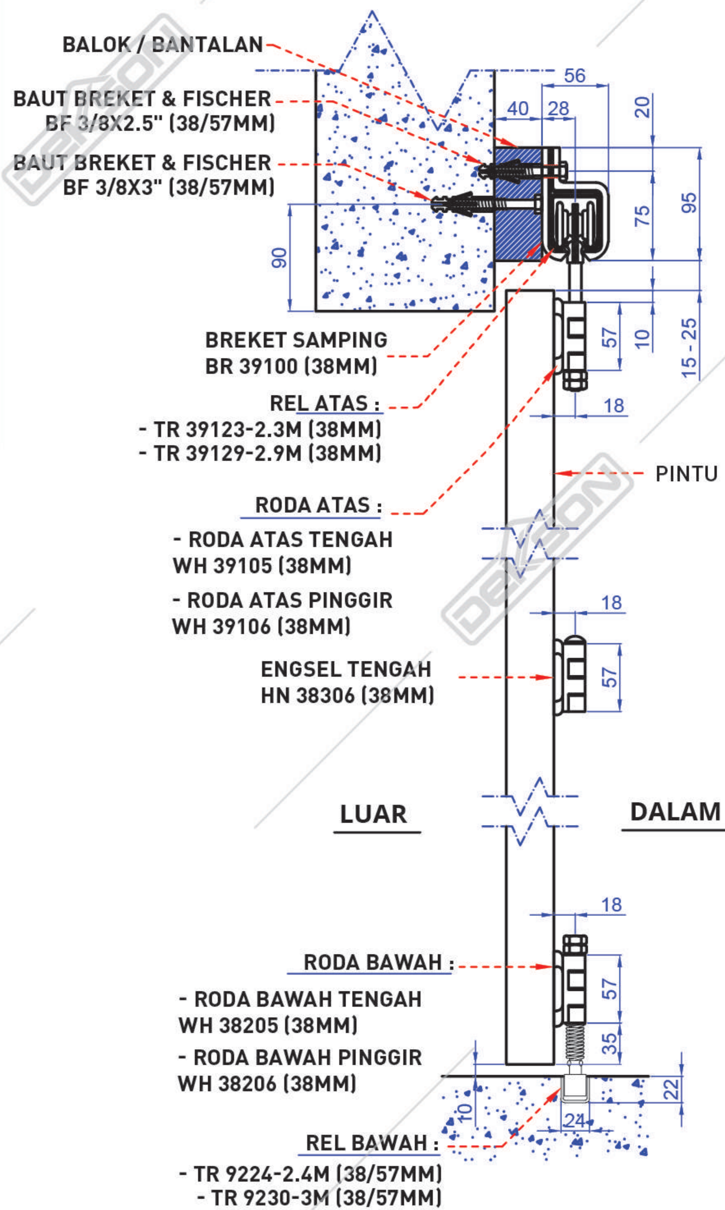
Gambar Potongan
