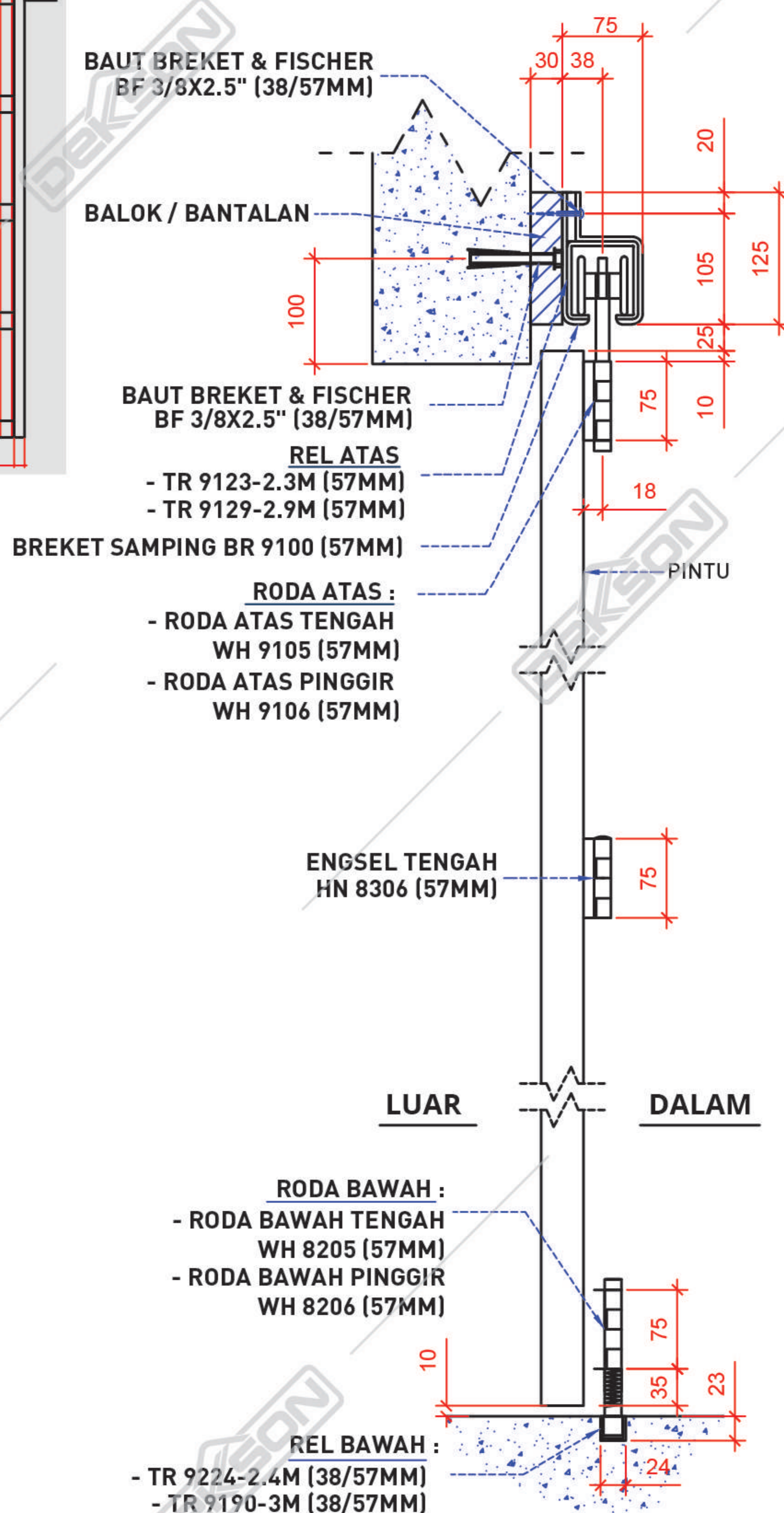
Gambar Potongan
