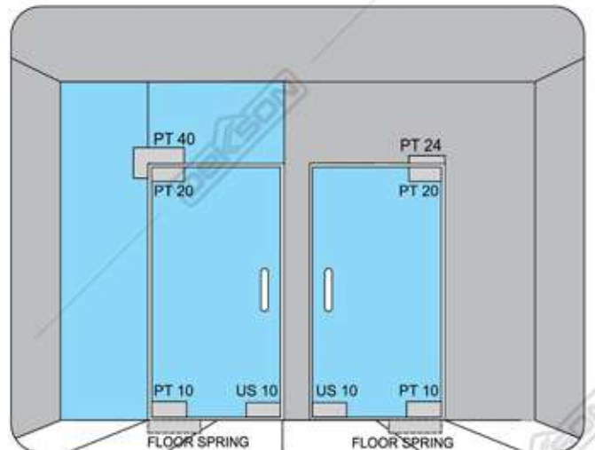
PTH 1080 PSS Glass Thickness : 8 - 12 mm Door Width : 800 mm (max) Door Weight : 80 Kg (max) FOR INDOOR USE
