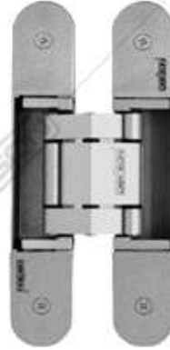
ES CONC 01 D80 NA Available : MATT BLACK Capacity (max) : 80 kg / pair Max. Door Width : 90 cm Opening Angle : \leq 150^\circ
